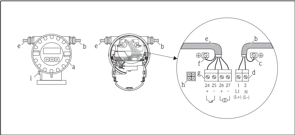
变送器的电气连接示意图 (现场铝外壳)，电缆横截面积：max. 2.5 mm² (14 AWG)
