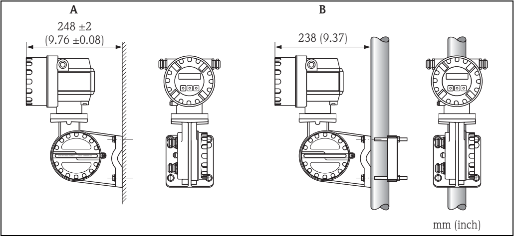
分体式仪表的变送器的安装示意图
