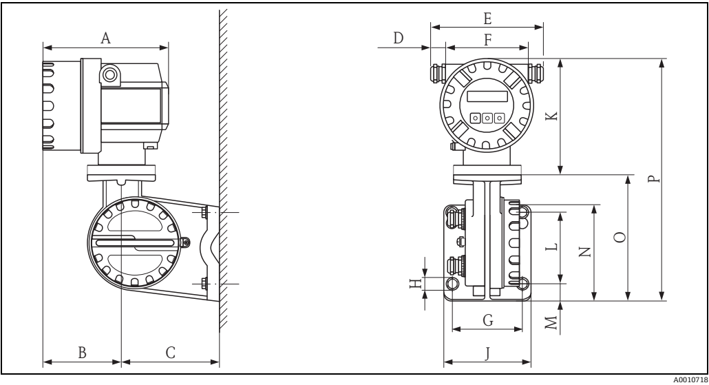
分体式仪表的变送器的外形尺寸示意图
