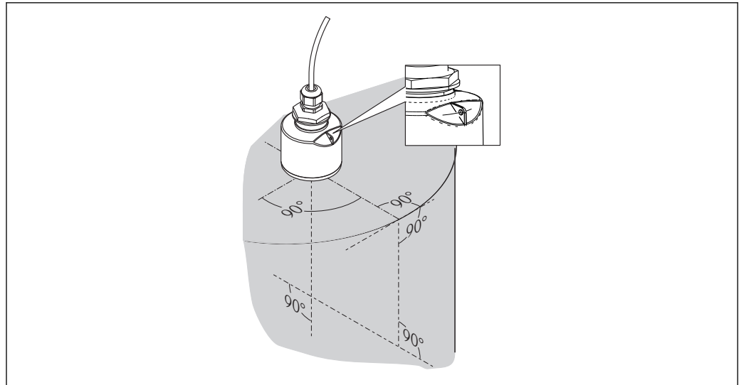
图 6 罐体中的传感器安装方向
