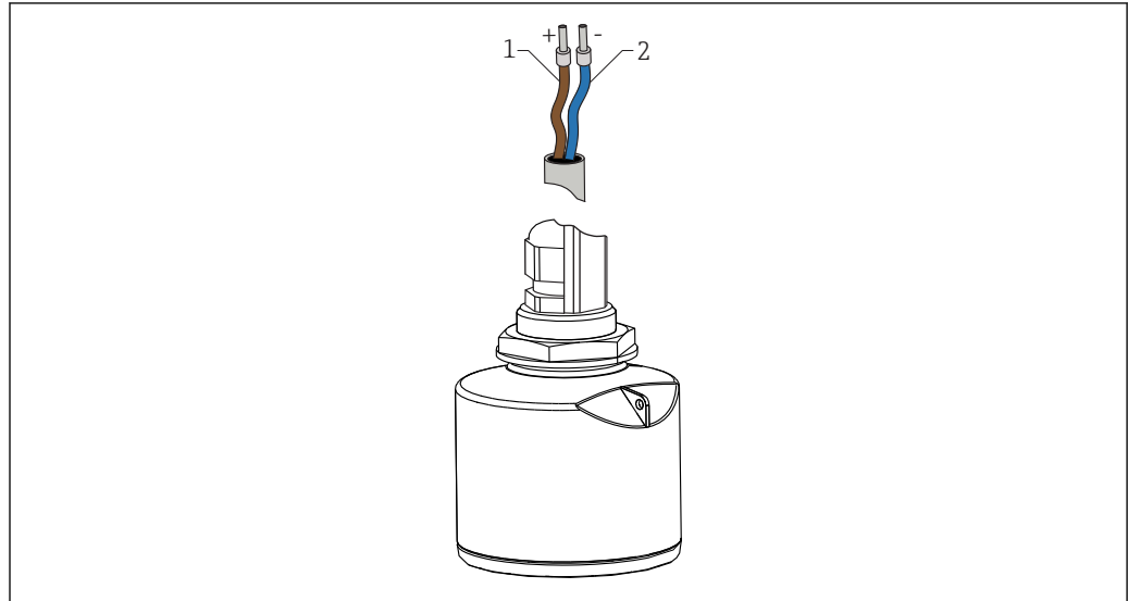
图 13 电缆分配
