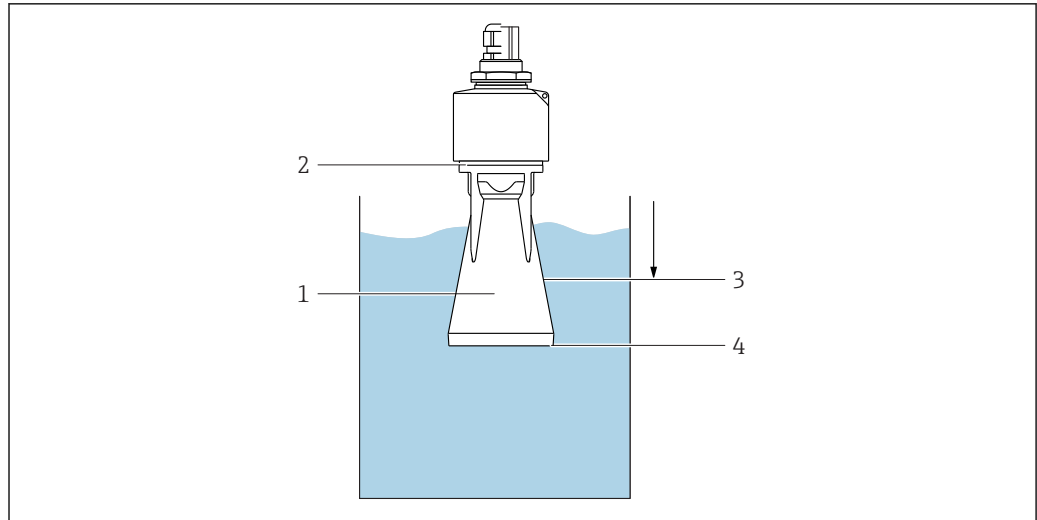
图 10 浸没罩功能示意图
