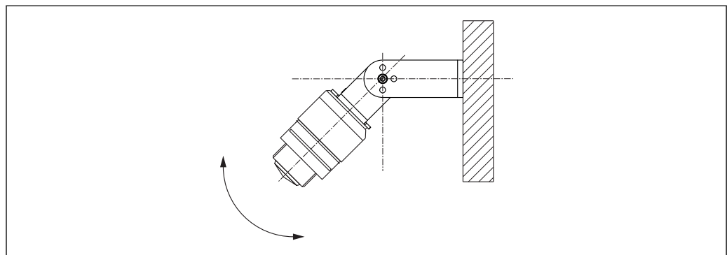
图 11 使用安装支架安装(可调节)
