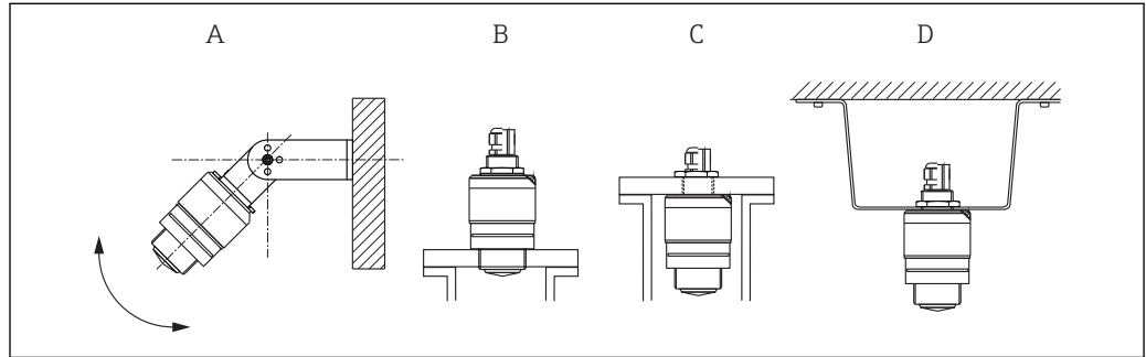
图 3 壁式安装、罐顶安装或安装短管安装
