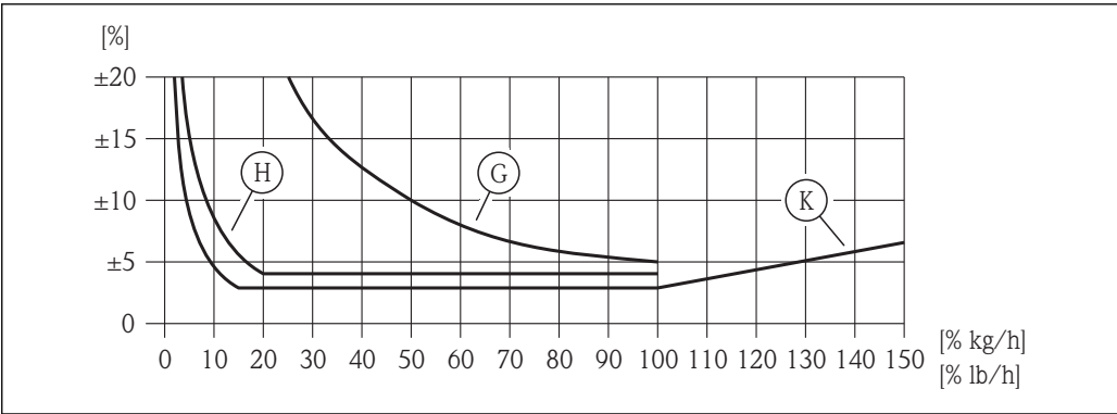
图 6 最大测量误差(%质量流量), 对应测量值/满量程值的%。订购选项“标定流量”, 选型代号 G、H、K; 请参考下表
