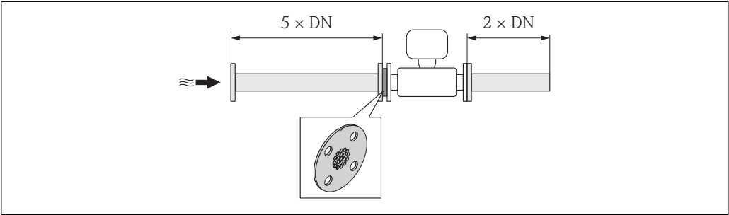
6 使用流量调节器时的推荐前后直管段长度
