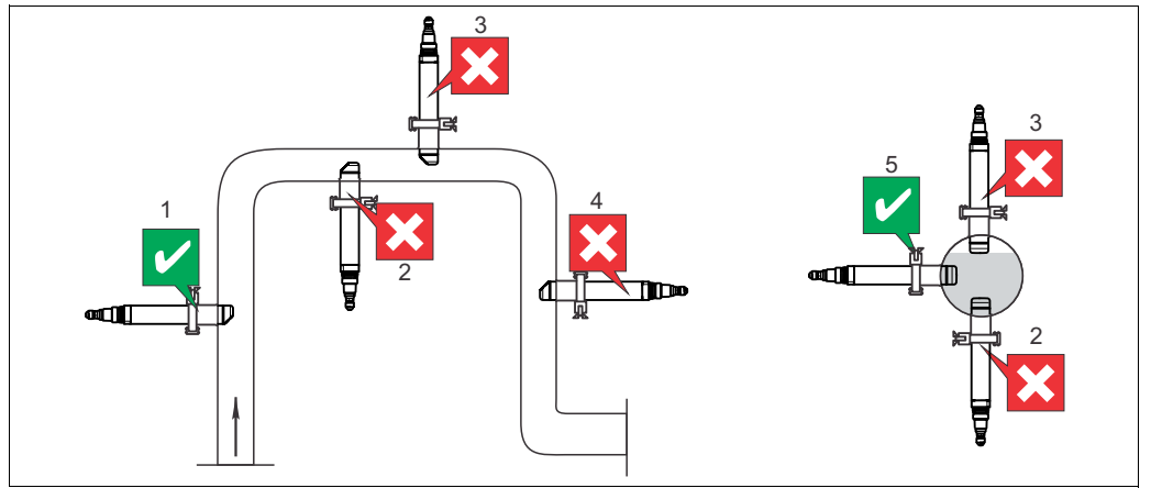
安装方向和安装位置示意图
