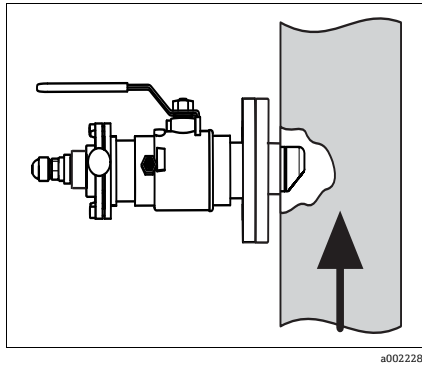
使用可伸缩式安装 CUA451 安装
