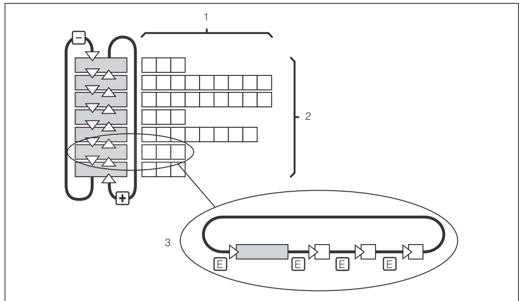
图 19 菜单结构示意图
