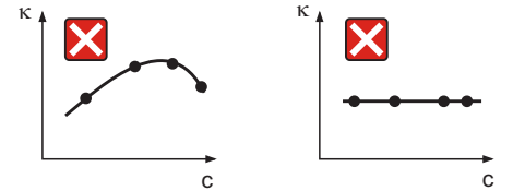
图 38 不允许出现的曲线
