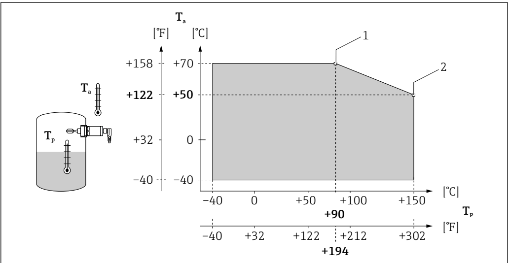
6 减温曲线: 150 °C (302 °F) 1 I max : 200 mA (DC-PNP), 250 mA (AC/DC) 2 I max : 150 mA (DC-PNP), 150 mA (AC/DC) Ta 环境温度范围 Tp 过程温度
