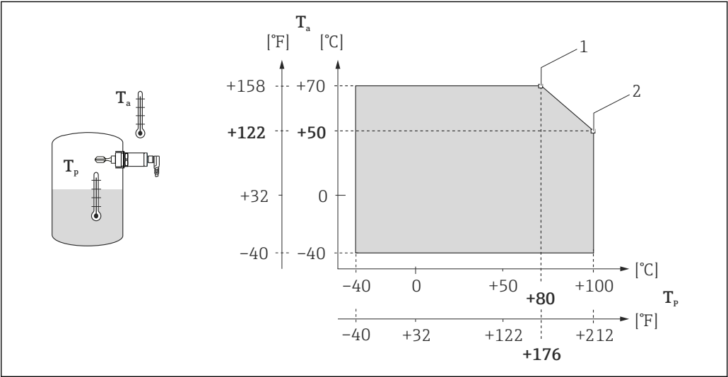
5 减温曲线: 100 °C (212 °F) 1 I max : 200 mA (DC-PNP), 250 mA (AC/DC) 2 I max : 150 mA (DC-PNP), 150 mA (AC/DC) Ta 环境温度范围 Tp 过程温度
