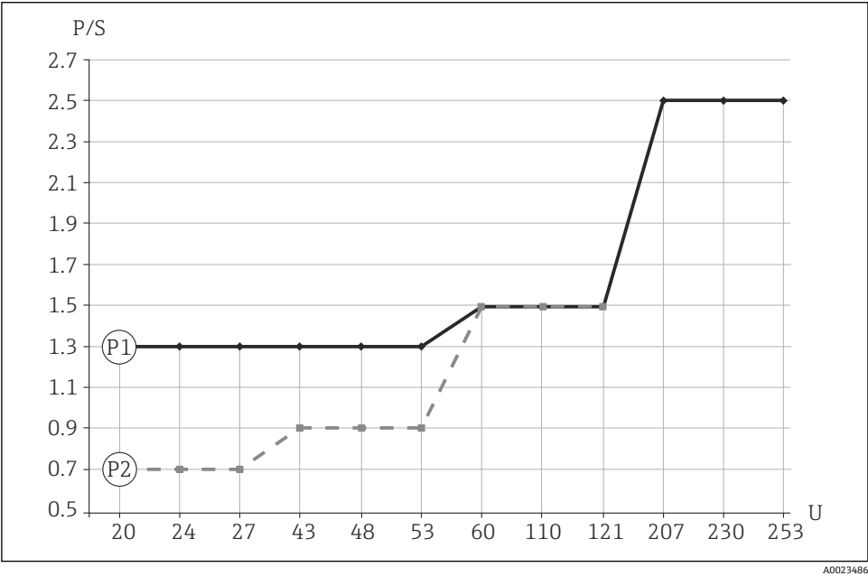
图 9 负载的最小额定功率
