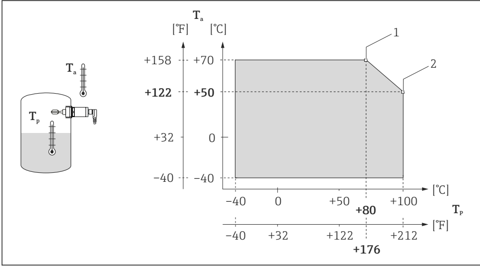
图 11 温度曲线: 100 °C (212 °F)
